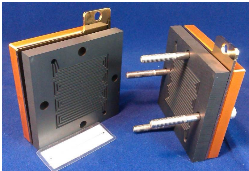
圖二:強固型單電池打開的樣子
