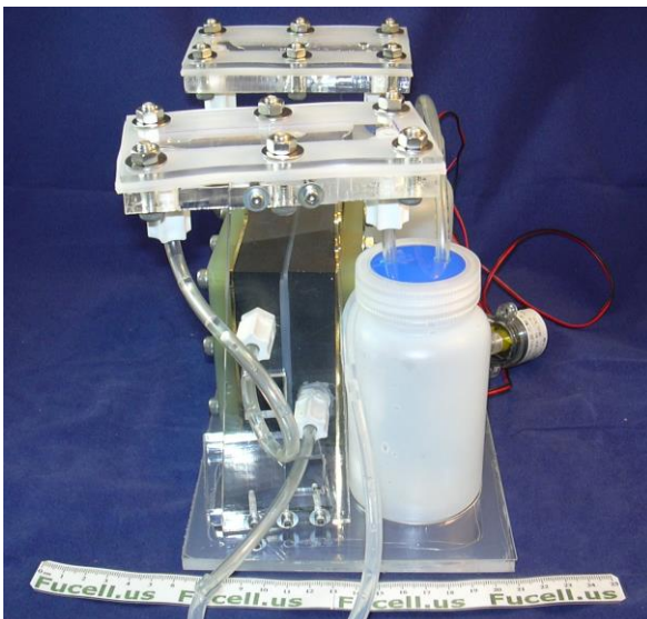
產品照片(三)：
